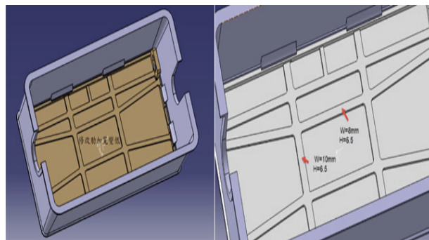
圖 12 40 型水量計箱結構優化#2
