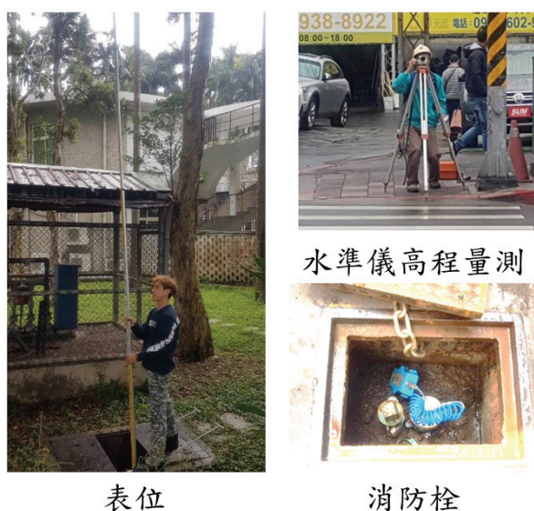
圖 5 表位、消防栓水準儀高程量測
