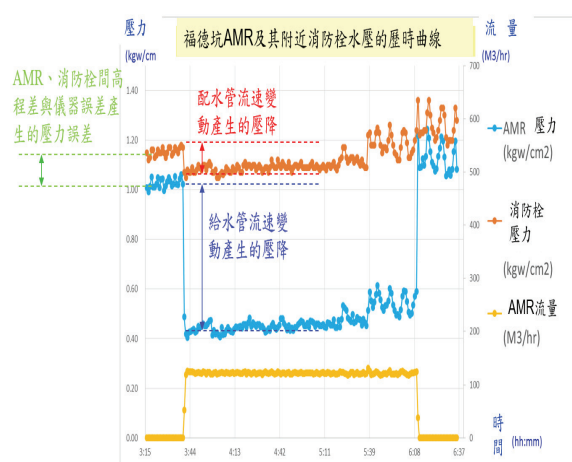
圖 6 因用戶大量進水產生配水管壓降案例
