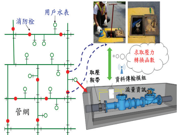
圖 1 實驗配置
