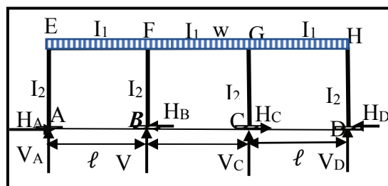
圖 3 剛架各梁柱之指數圖
