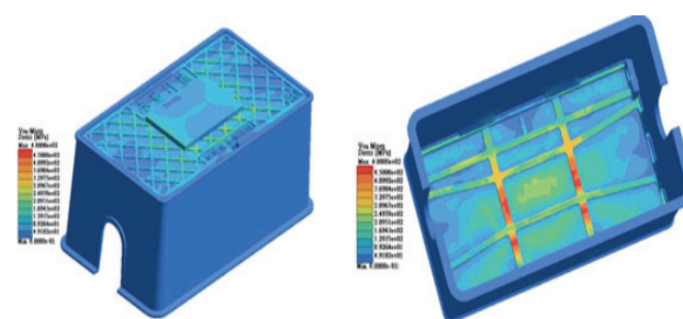
圖 13 40 型水量計箱結構優化#2 應力分析
